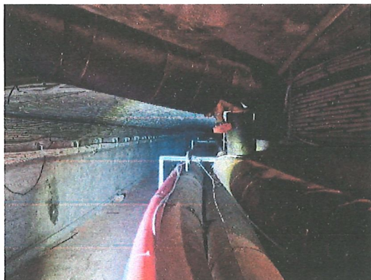
#1 Oversigt installationsgang.
