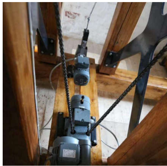
Automatisk ringning og jern kryd mellem lodrette stolper i klokkestol. Fra en anden kirke.
