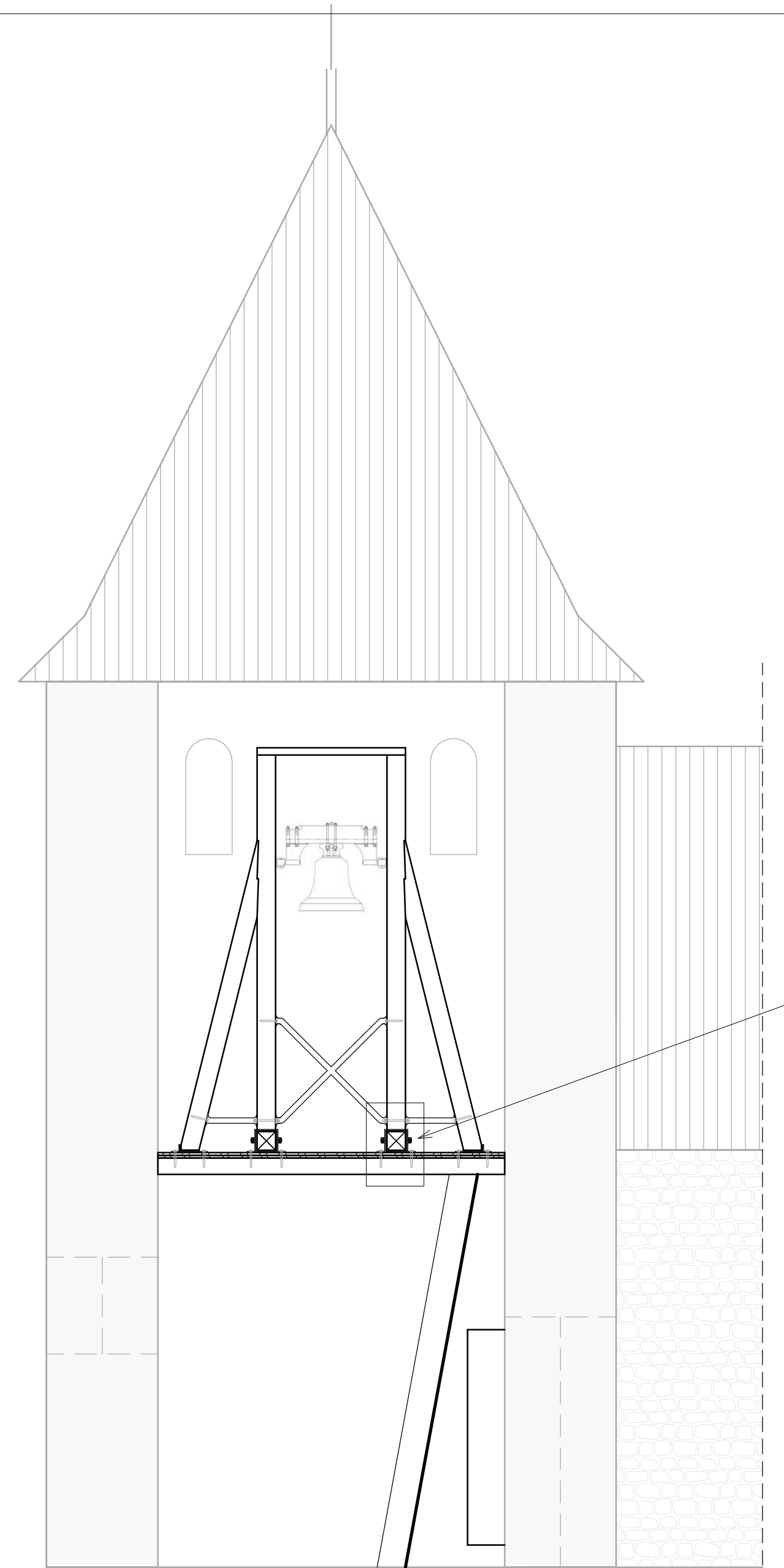
Snit i tårn set fra syd.
