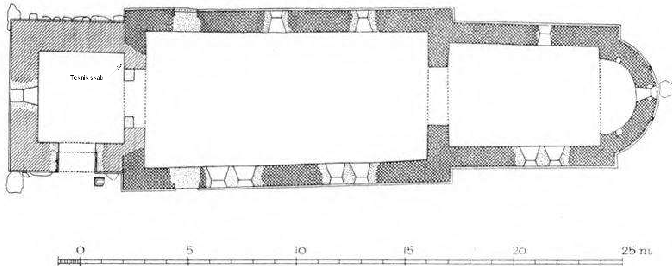
Fig. 2. Vejerslev. Plan. 1:300. Maalt af C. G. Schultz 1939.
