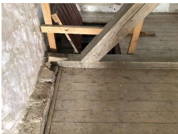
Klokkestolens lejebjælker ligger af på loftets bjælker, loftet er gennembrudt.
