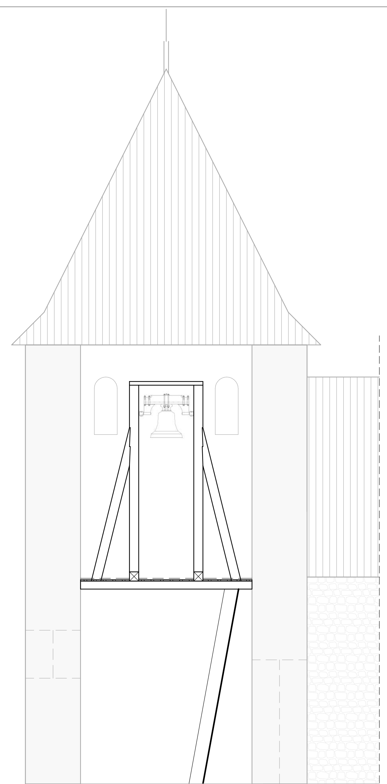
Snit i tårn set fra syd.
