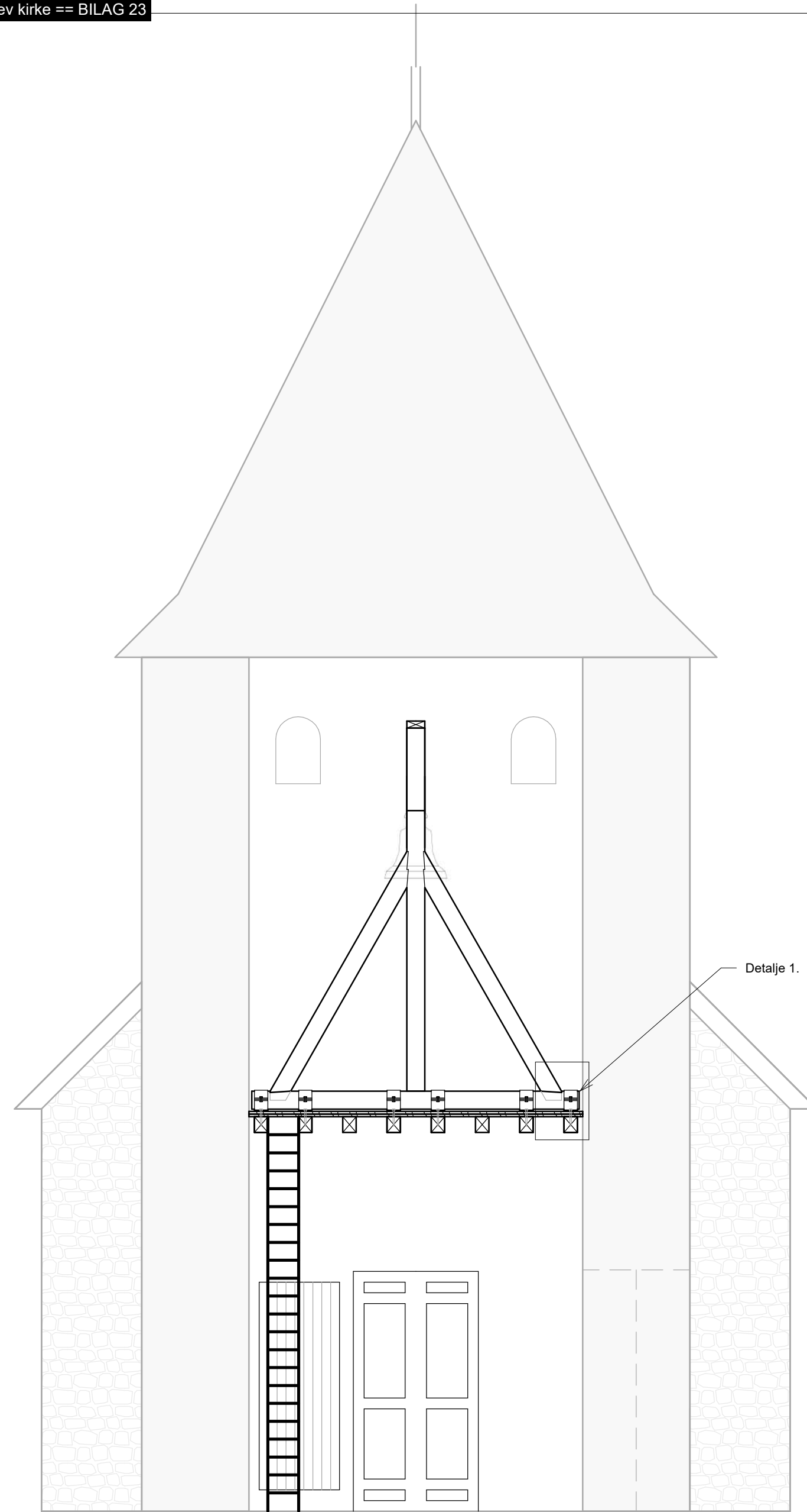
Snit i tårn set fra vest
