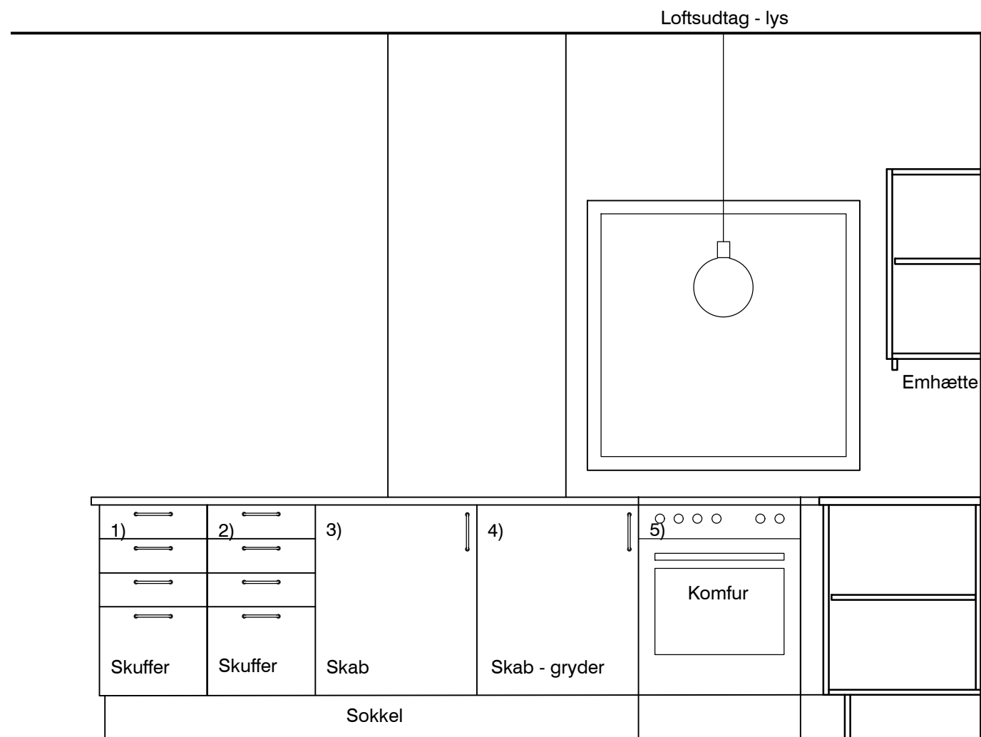
SNIT A-A
